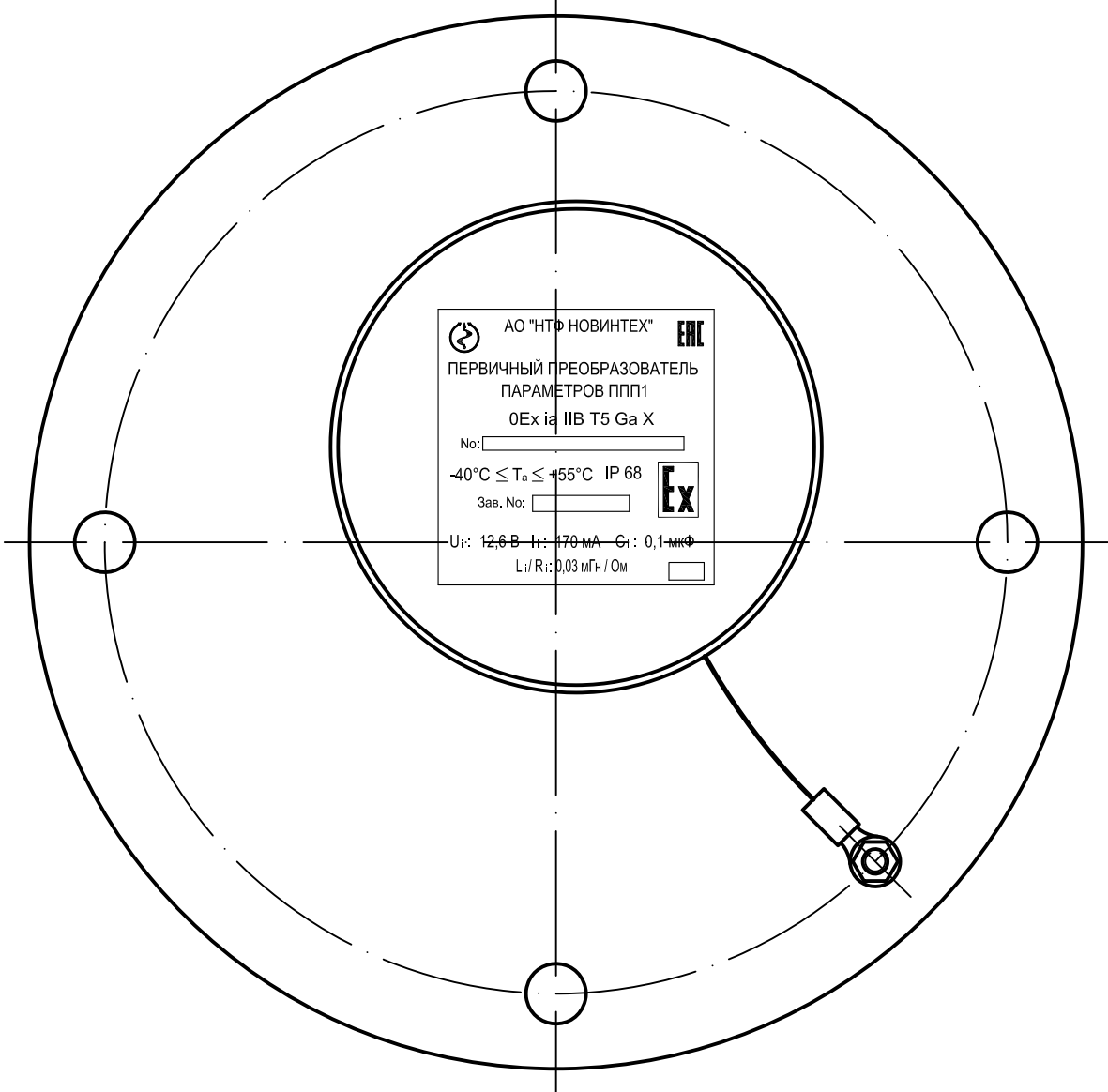
Вид сверху 1:1
