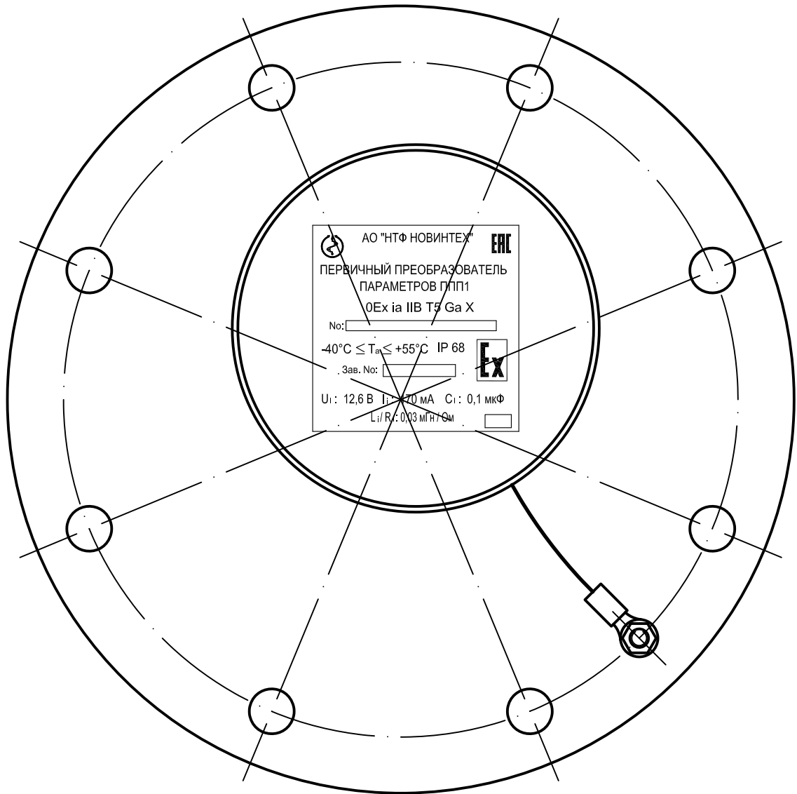
Вид сверху 1:1 (вариант с фланцами из нержавеющей стали)
