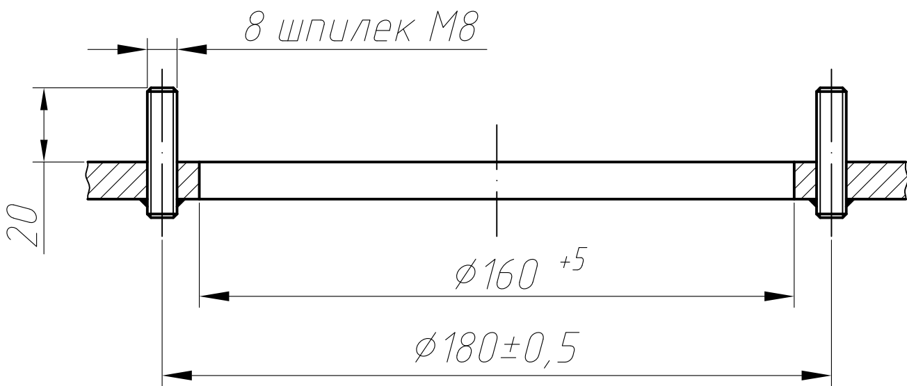
Посадочное место 1:1 (вариант с фланцами из нержавеющей стали)
