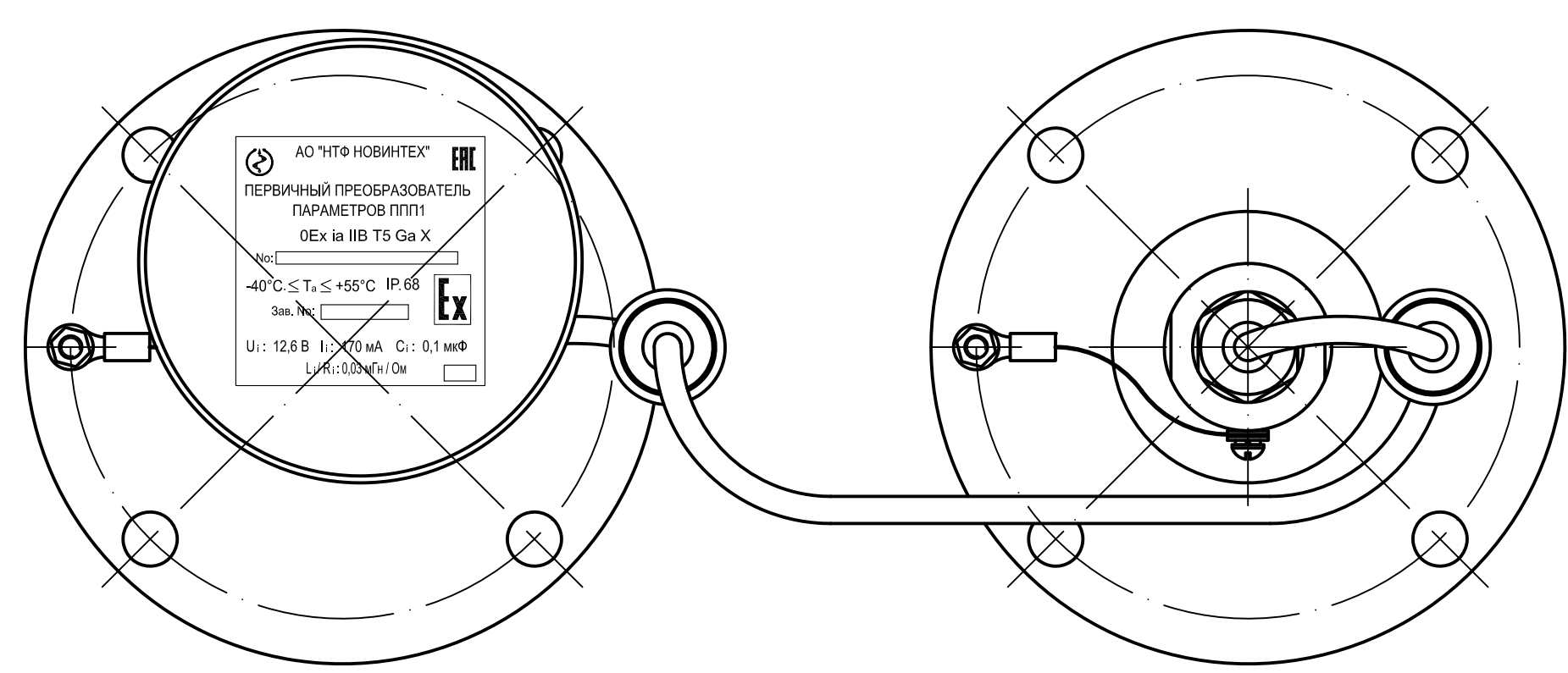
Вид сверху 1:1
