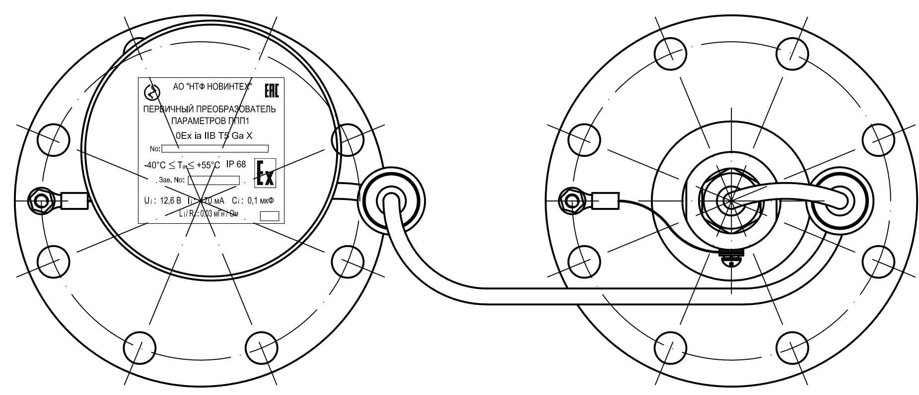
Вид сверху 1:1 (вариант с фланцами из нержавеющей стали)
