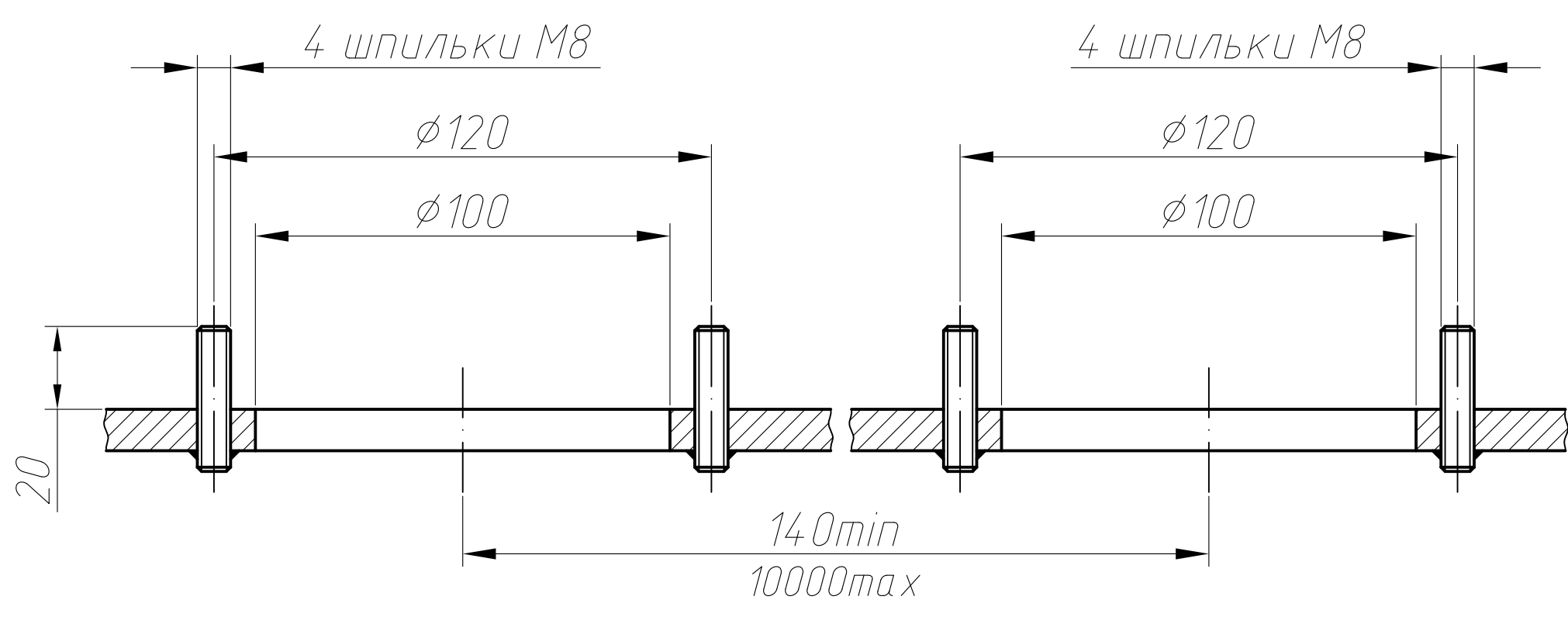
Посадочное место 1:1
