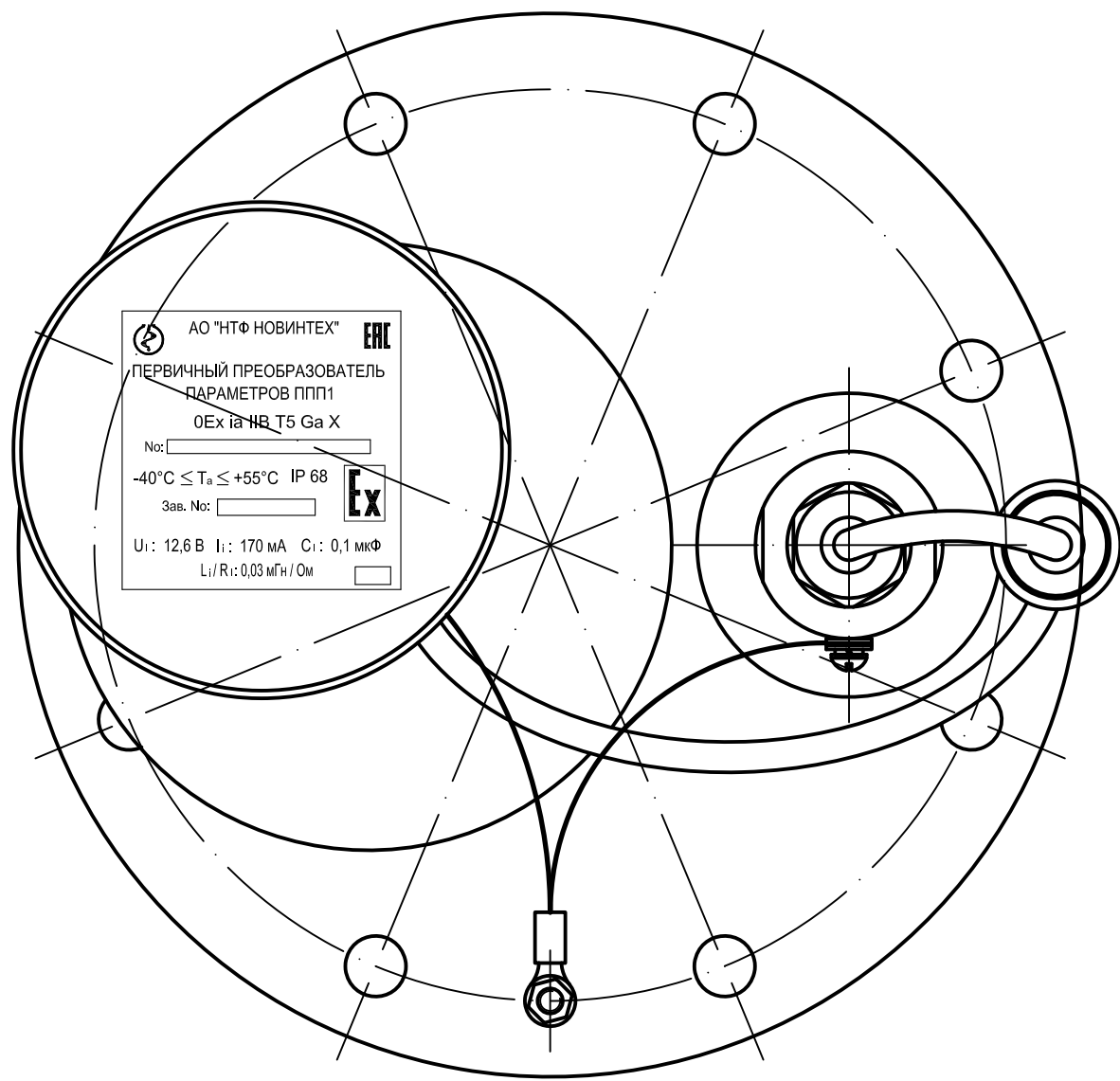
Вид сверху 1:1 (вариант с фланцами из нержавеющей стали)
