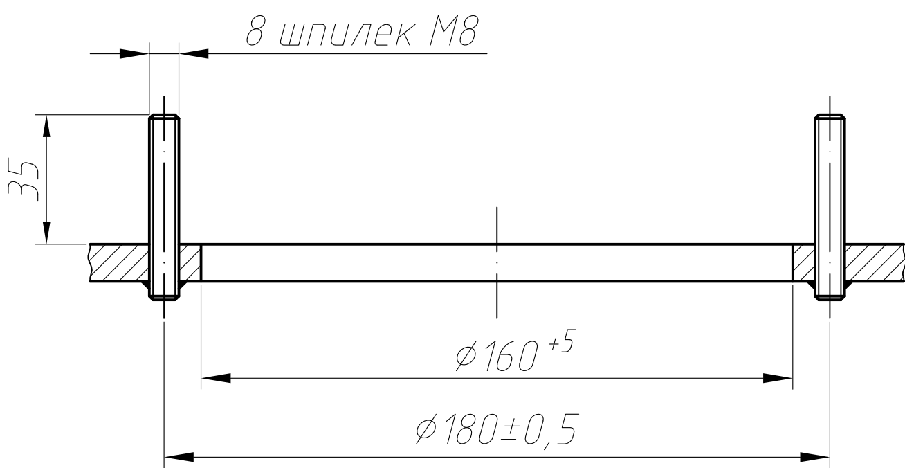
Посадочное место 1:1 (вариант с фланцами из нержавеющей стали)
