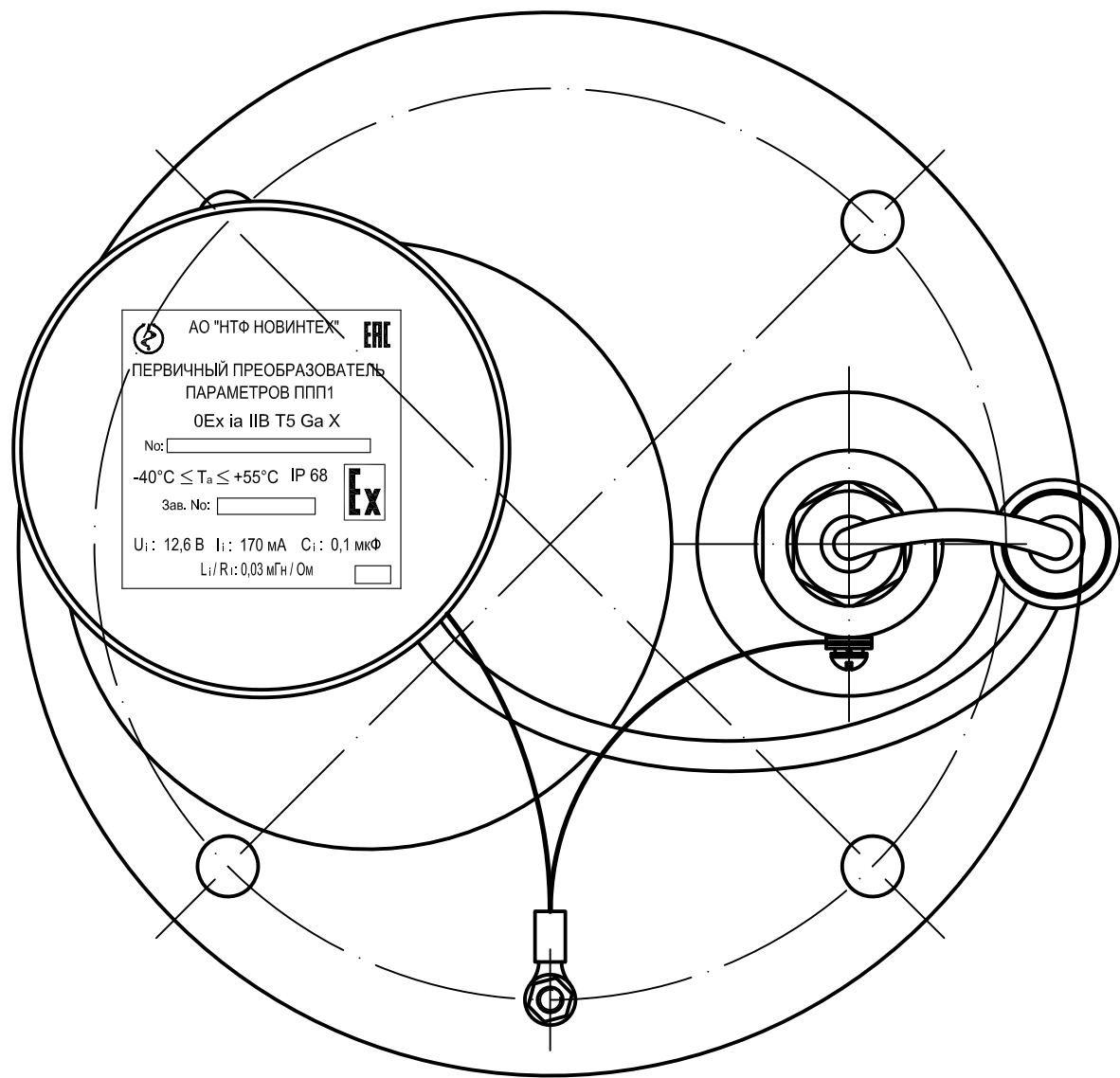
Вид сверху 1:1
