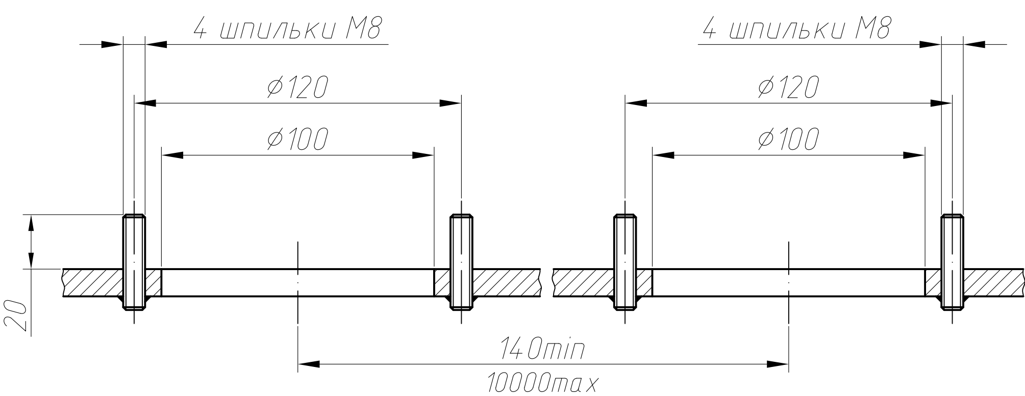
Посадочное место 1:1
