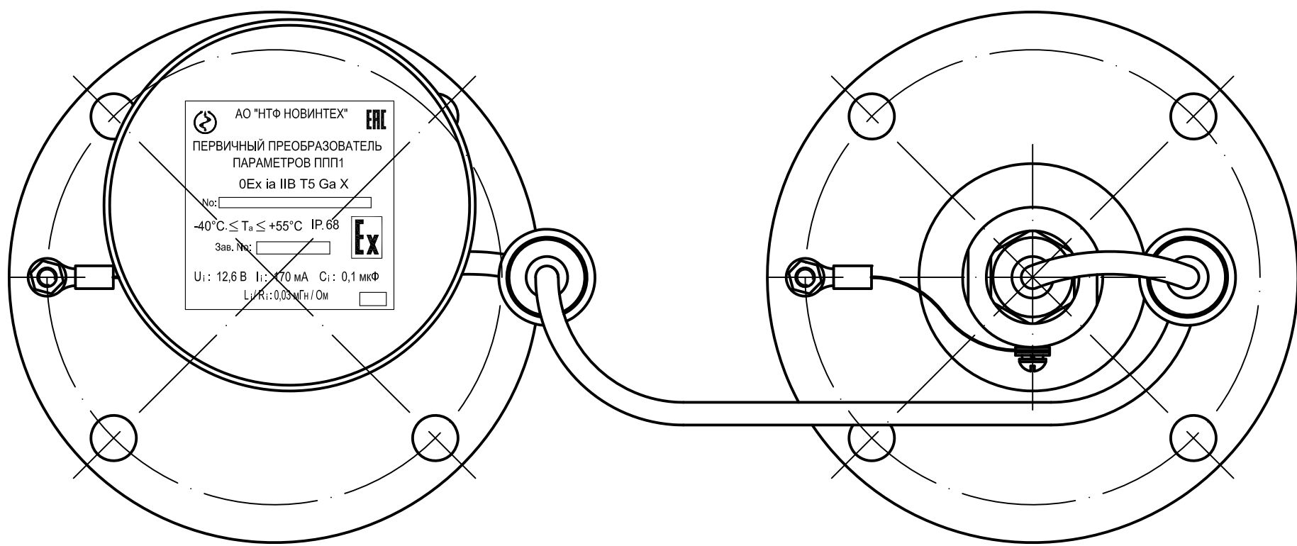
Вид сверху 1:1
