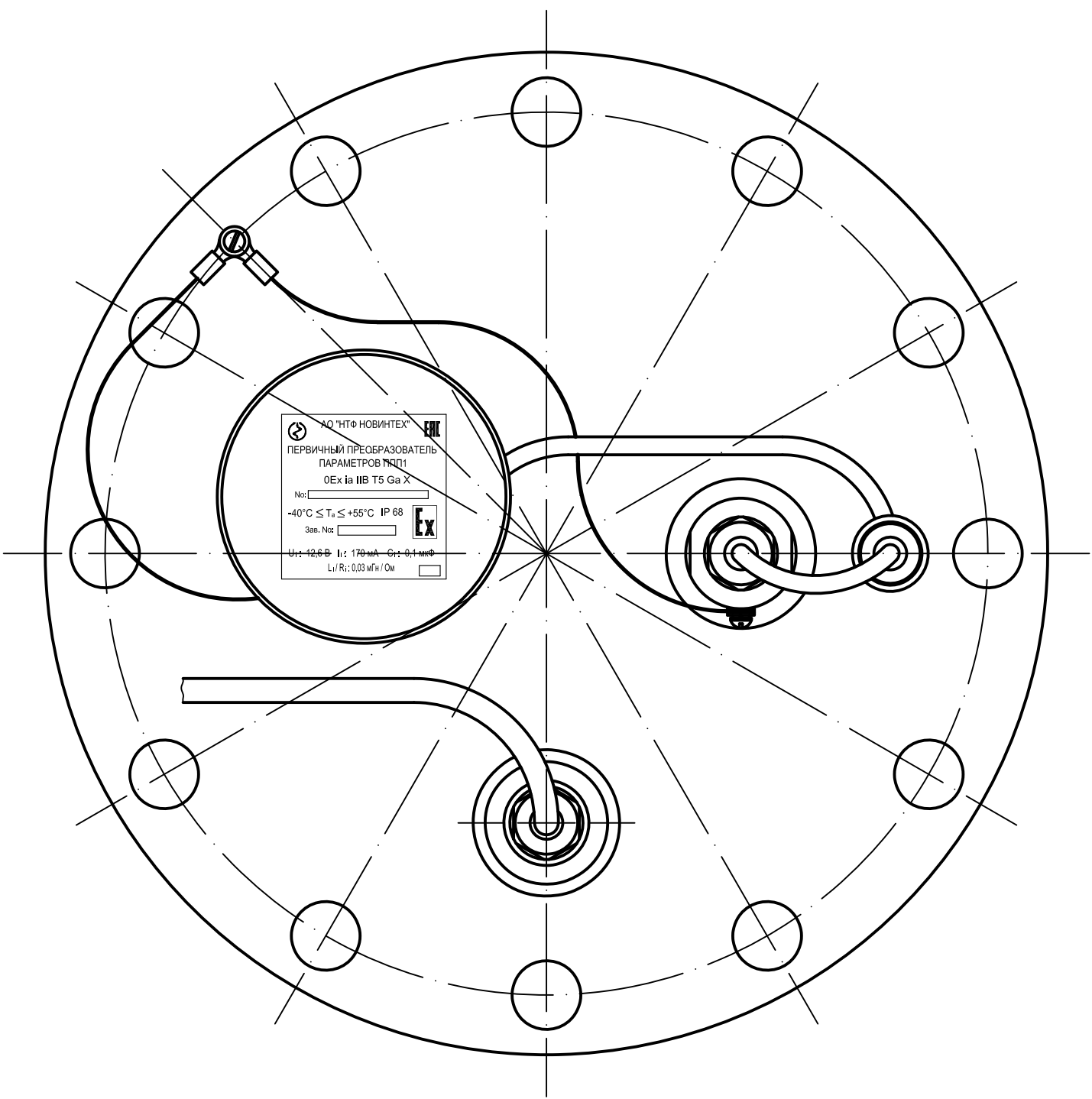
Вид сверху 1:1
