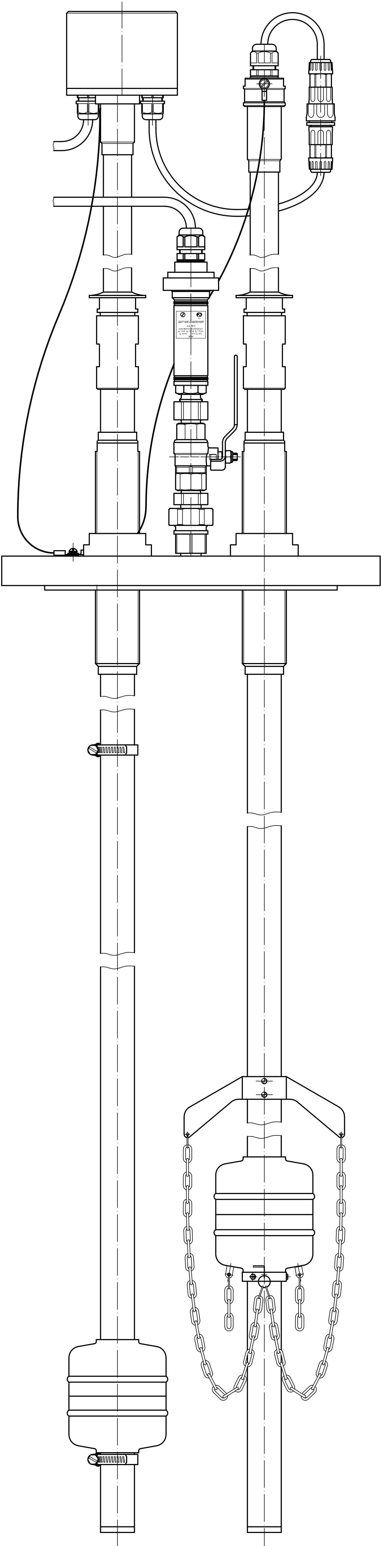
Главный вид 1:1
